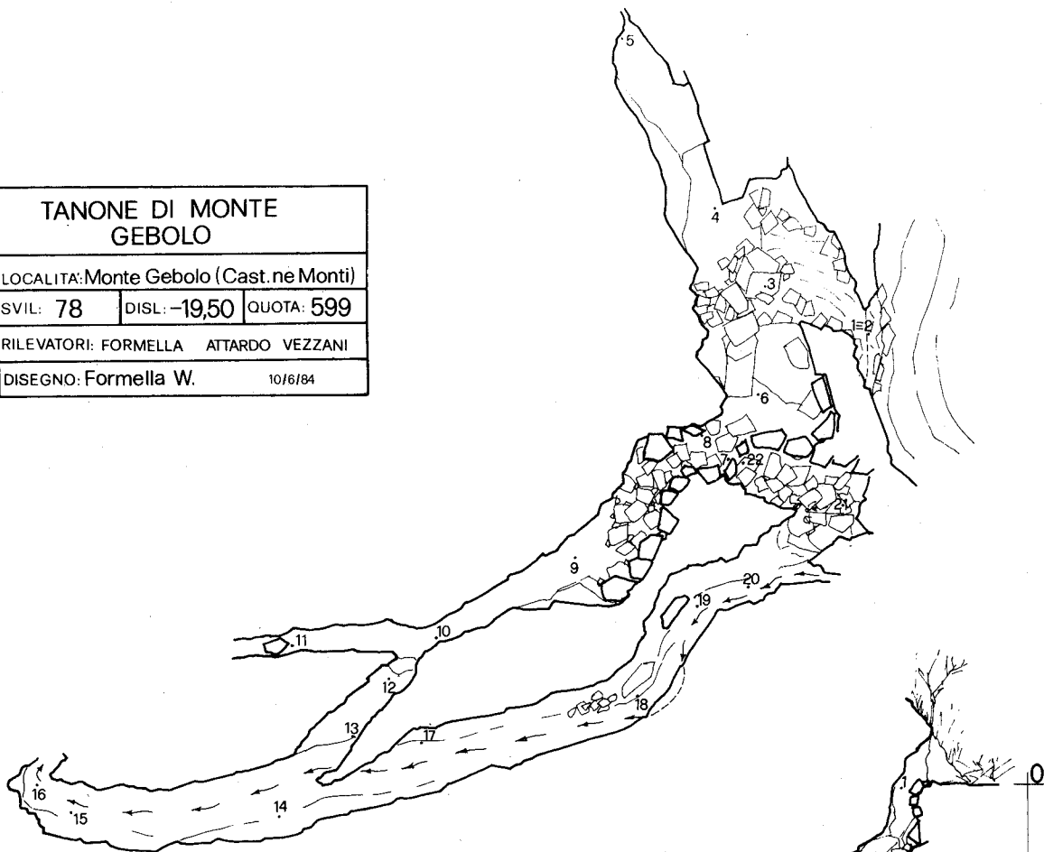
PIANTA
